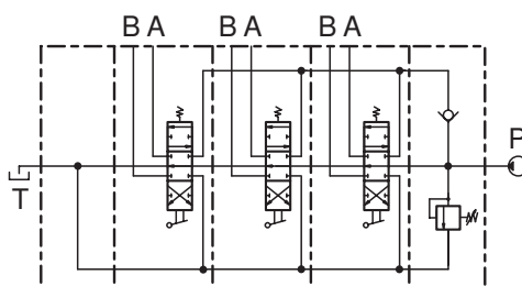
HYDRAULIC SCHEMA - SCHEMA IDRAULICO
