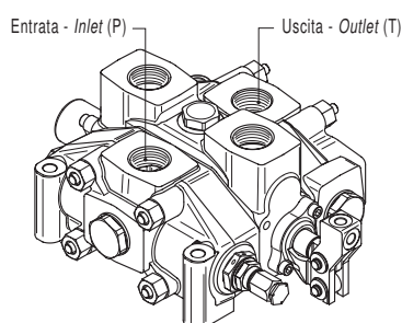
LEFT INLET SECTION COLLETTORE ENTRATA SINISTRA
