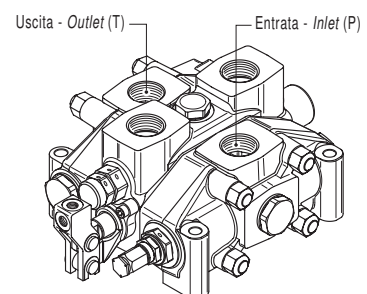
RIGHT INLET SECTION COLLETTORE ENTRATA DESTRA
