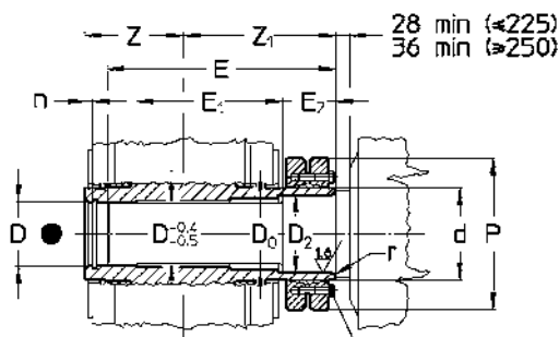
c) Albero lento cavo differenziato con unità di bloccaggio e perno macchina «lungo» c) Stepped hollow low speed shaft with locking assembly and «long» machine shaft end
