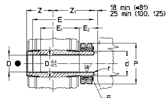
a) Albero lento cavo con unità di bloccaggio e perno macchina. a) Hollow low speed shaft with shrink disc and machine shaft end.
