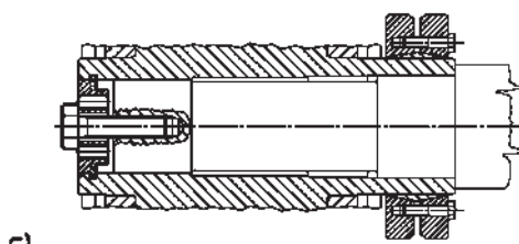
Calettamento con unità di bloccaggio c) Fitting with shrink disc c)
