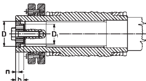
Calettamento con unità di bloccaggio c) Fitting with shrink disc c)
