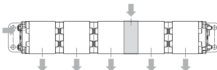
5 sezioni con 2 ingressi: laterale e posteriore con collettore 5 sections with 2 inlets; side and rear with collector
